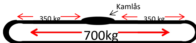
Figur 1: Förbandsinstallation draghållfasthet, minimum brottlast
